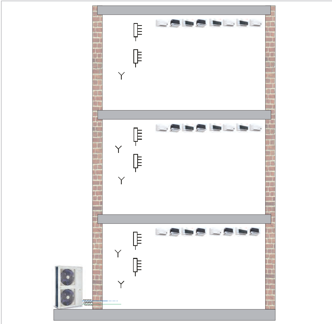
Abb. 17: Skizze zur Ermittlung der nachzufüllenden Kältemittelmenge
