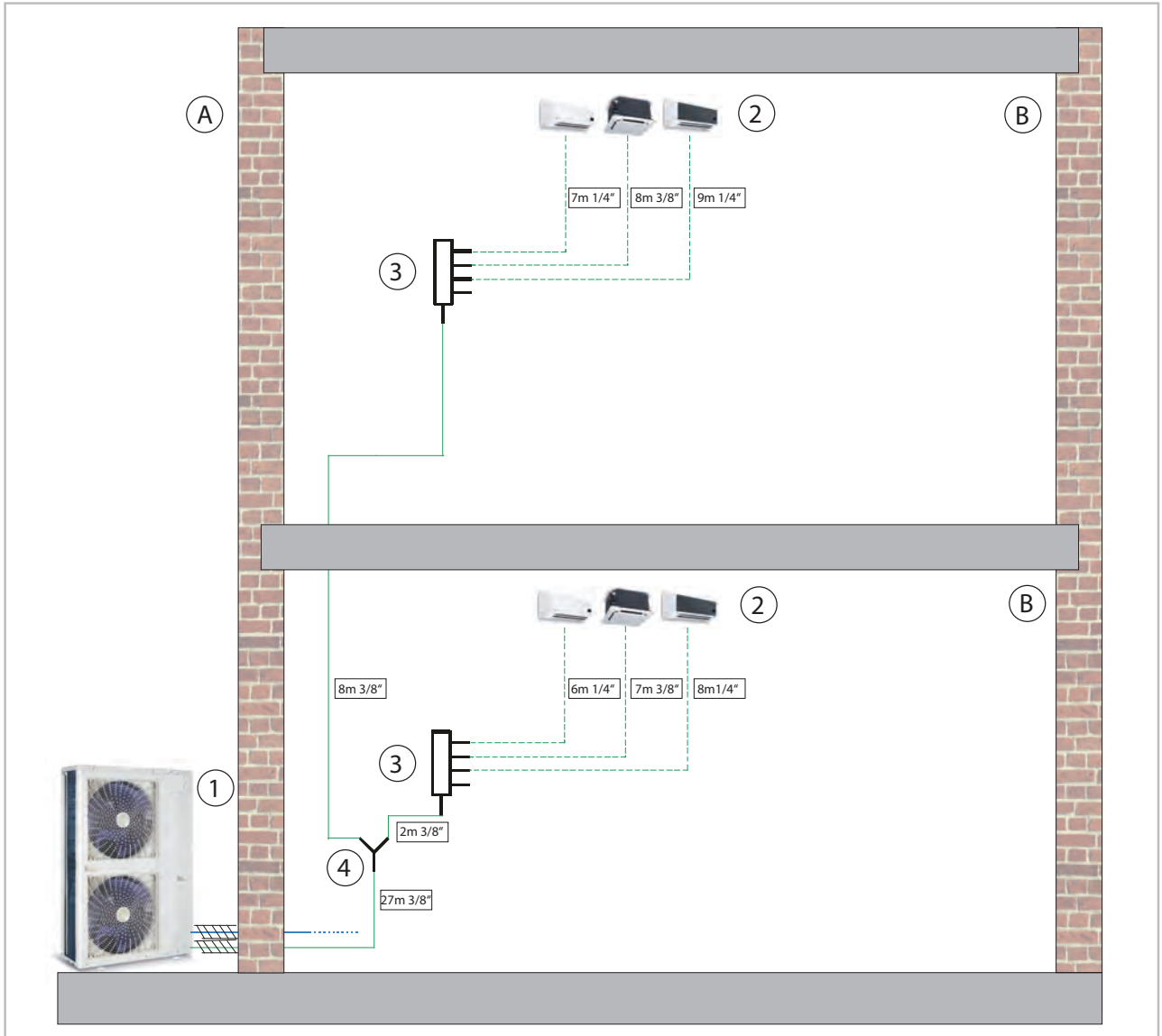
Abb. 16: Beispielkombination für die Berechnung der Kältemittelzusatzfüllung
