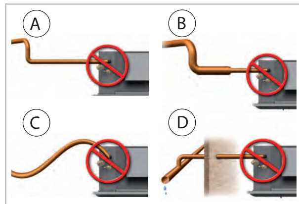
Abb. 18: Kondensatanschluss - Falsch!
