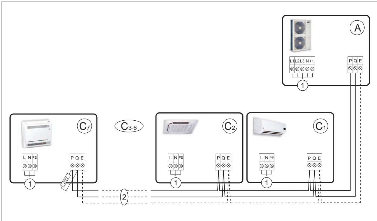
Abb. 22: Elektrisches Anschlussschema
